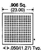
Footprint 225-2
