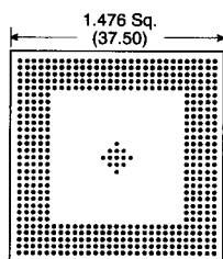
Footprint 493
